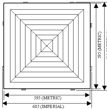
(ST-60) TEEBAR
